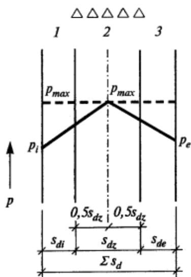
Фиг. 6.5б. Дифузия на водната пара по време на изпаряването след кондензационен пад във вътрешността на ограждащата конструкция или елемент
