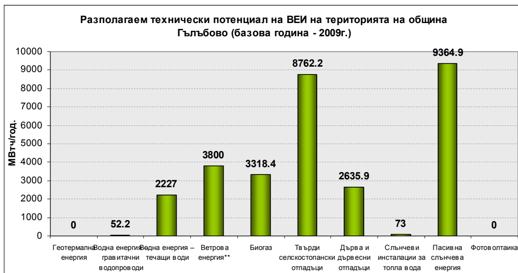
Фигура 6. Технически потенциал на ВЕИ.
